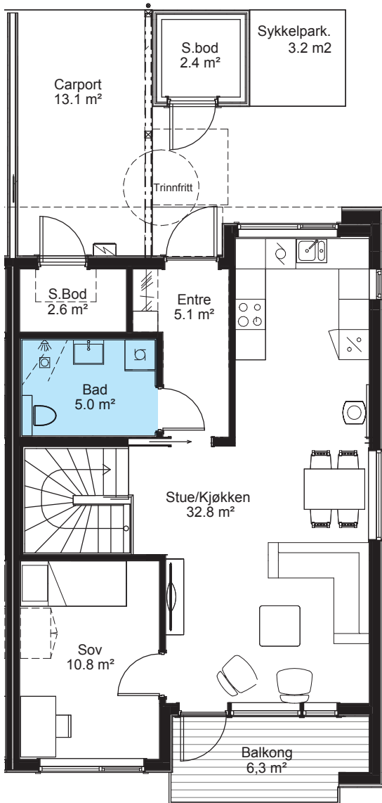
1. etasje
